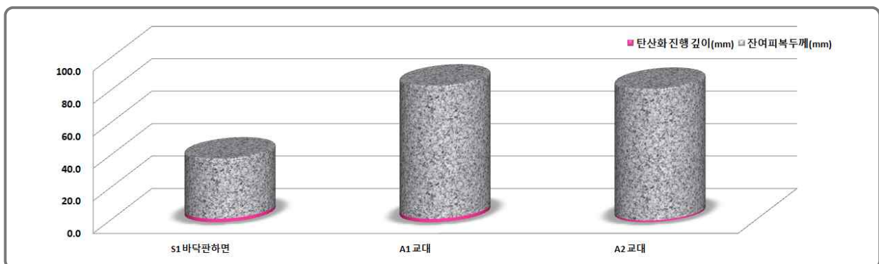
[그림 8.3.6] 탄산화깊이 및 잔여피복두께 측정결과
