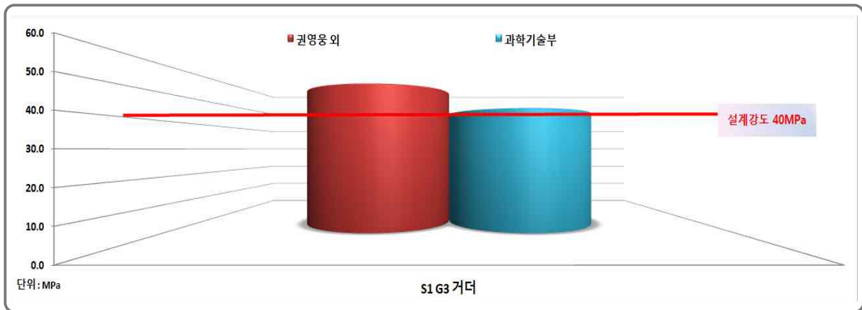
[그림 8.3.4] 반발경도법에 의한 비파괴강도 측정 결과-상부구조(거더)
