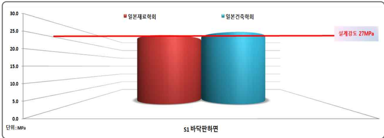
[그림 8.3.3] 반발경도법에 의한 비파괴강도 측정 결과-상부구조(바닥판하면)
