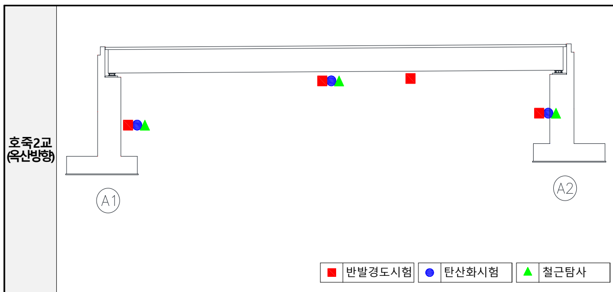
[그림 8.3.2] 비파괴시험 위치도
